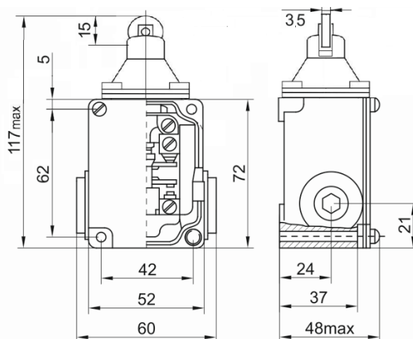
Рис.2. ВПК-2111-БУ2 - привод толкатель с роликом
